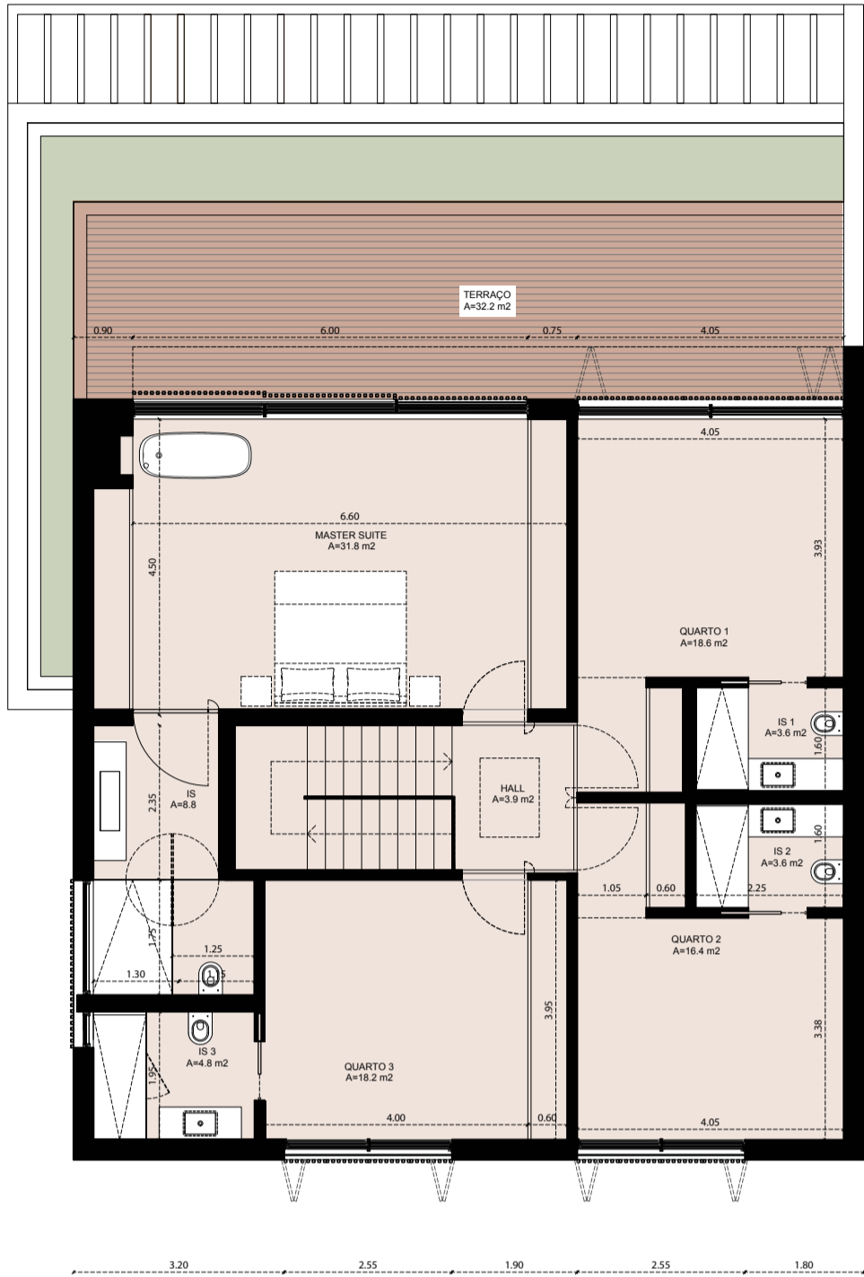
First floor | 1º piso
